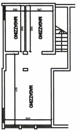
PIANTA INTERATO 1:100
